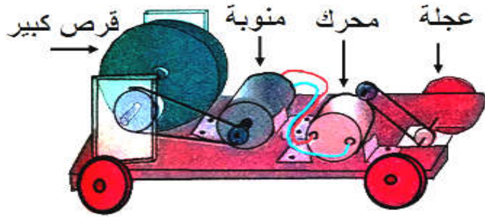
وثيقة 1 - عربة تتحرك ذاتيا
