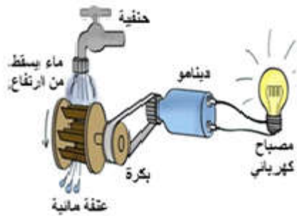
مصباح يشتعل بواسطة سقوط الماء من ارتفاع
